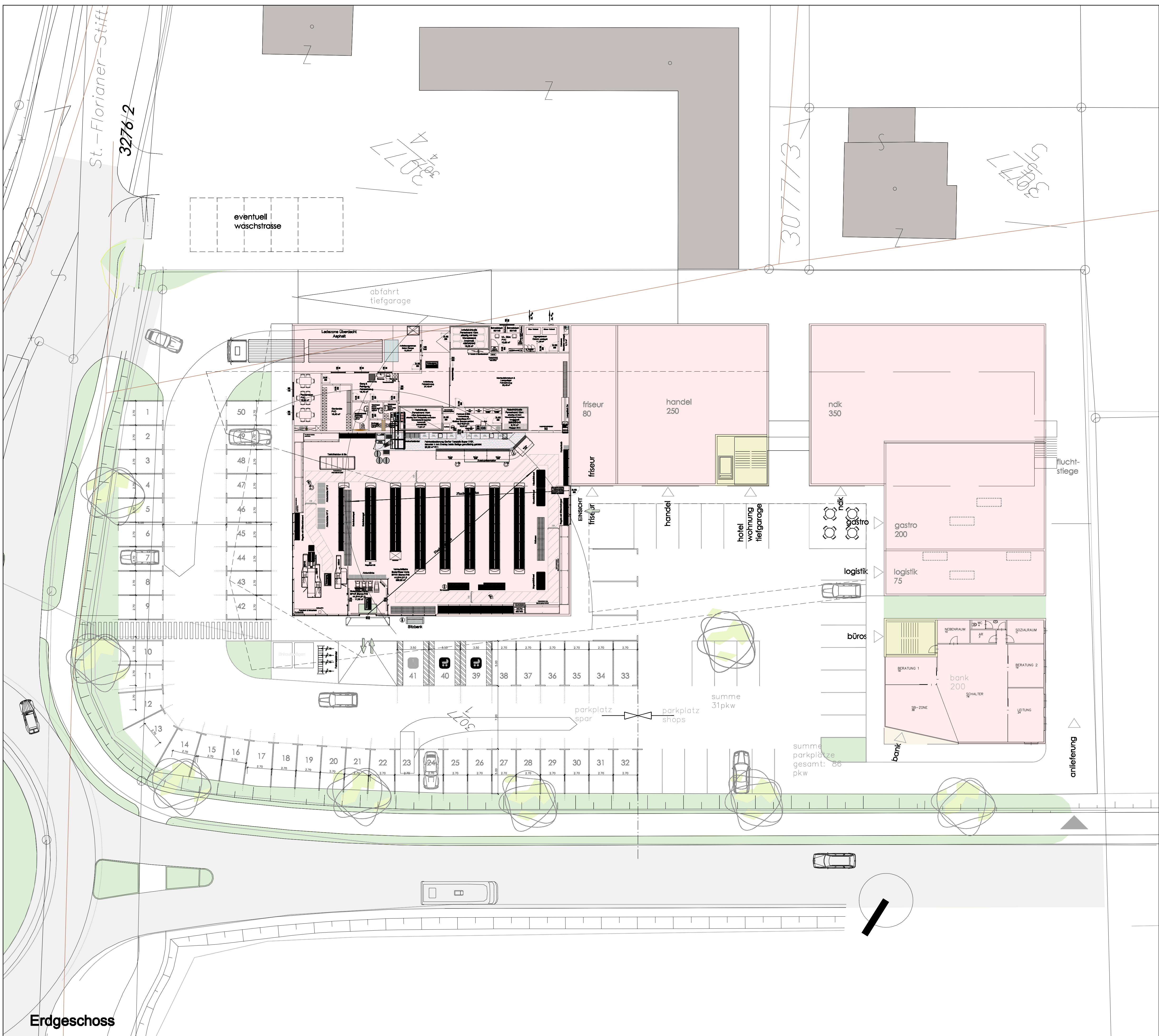
Lageplan M=1:1000
